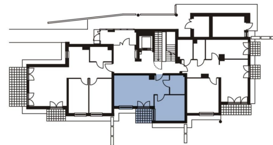
Rzut parteru
